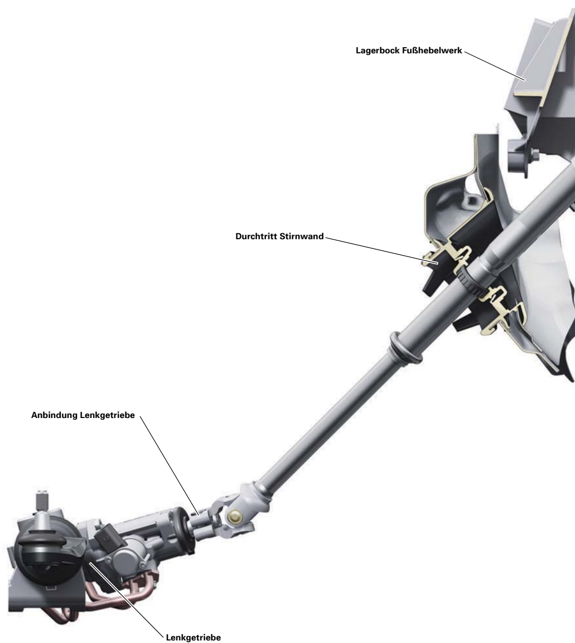
Schnittdarstellung der Lenksäule im eingebauten Zustand
