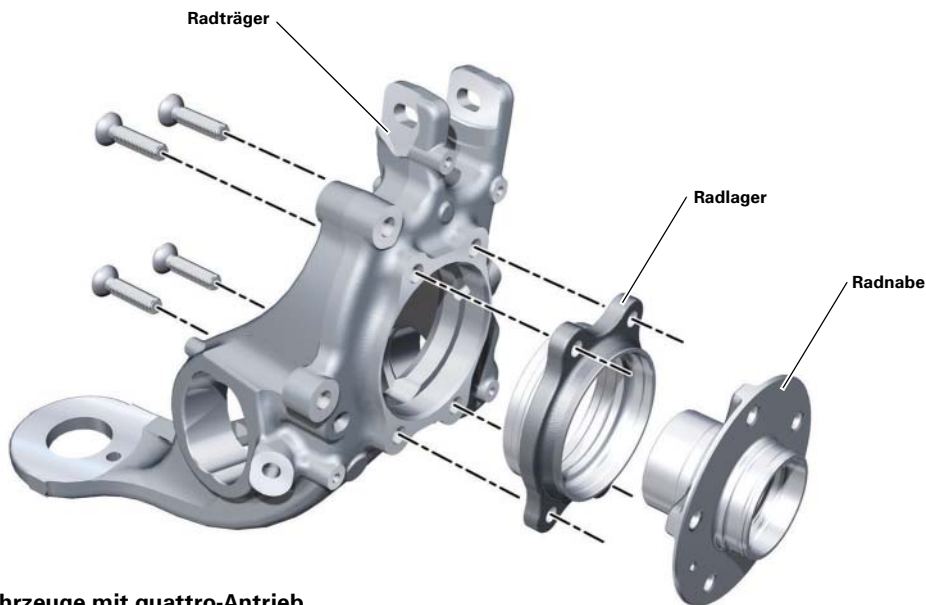
Radlagerung für Fahrzeuge mit quattro-Antrieb
