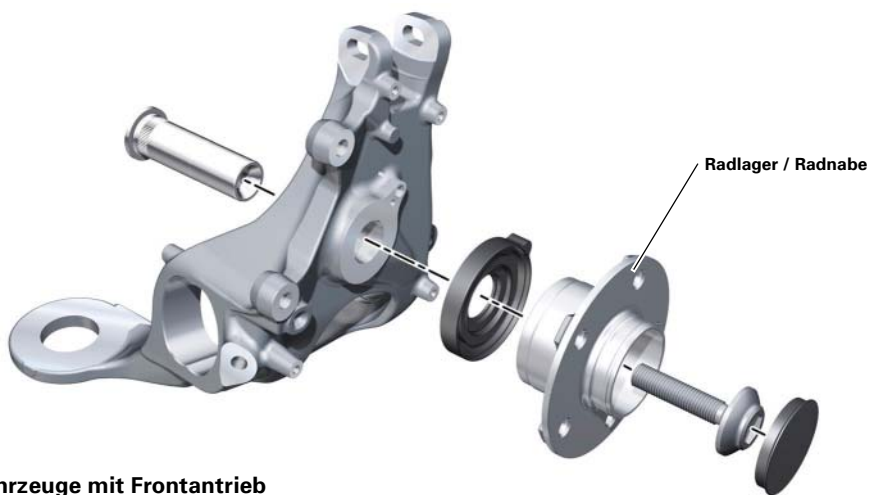
Radlagerung für Fahrzeuge mit Frontantrieb
